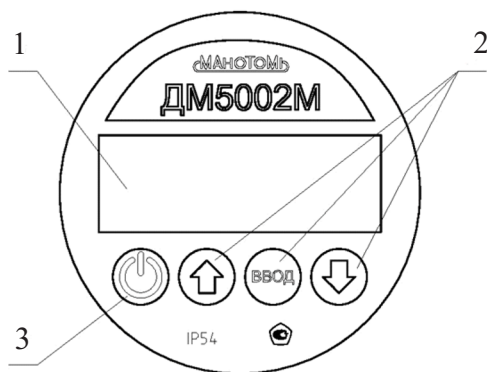
Рисунок 2.1 – Панель индикации ДМ5002М
