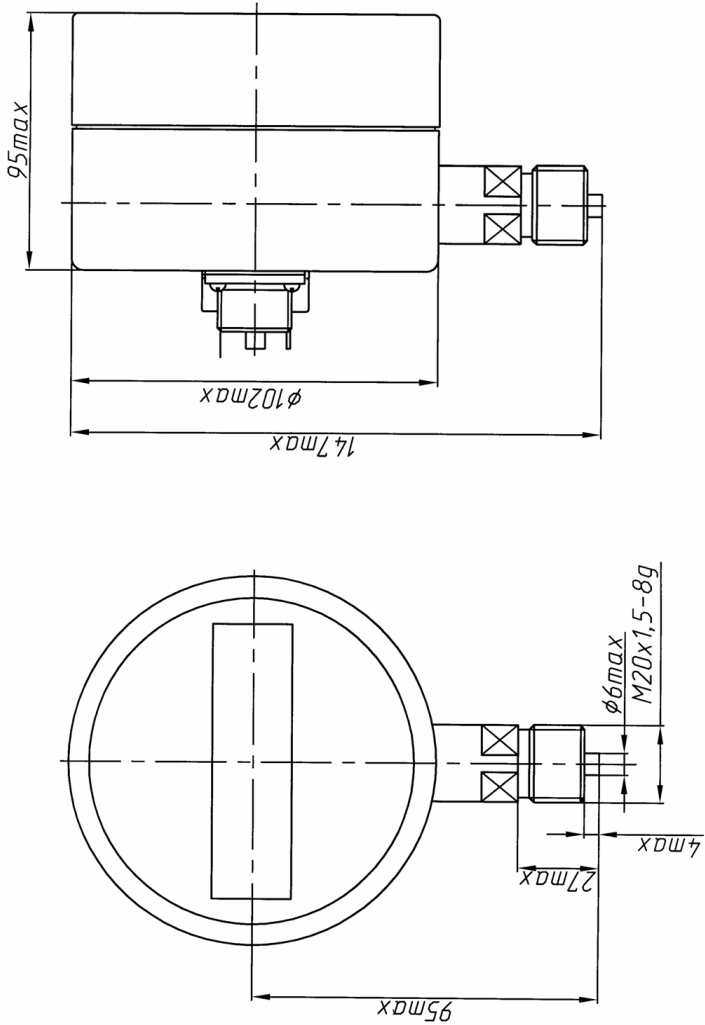
Рисунок Б.1 Габаритные и присоединительные размеры приборов ДМ5002М
